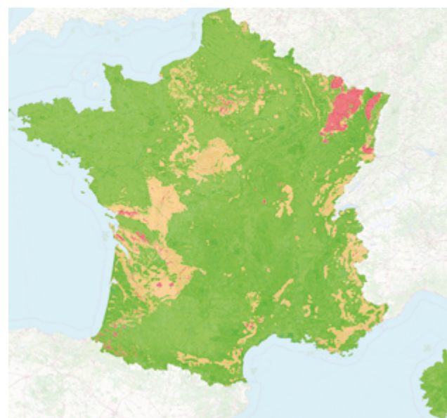
Carte réglementaire nationale de la géothermie de minime importance sur sondes géothermiques verticales à 200 m de profondeur
